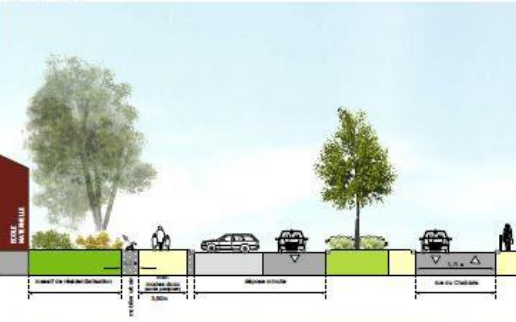
AA' COUPE DE PRINCIPE SUR LA DÉPÔSE MINUTE / STATIONNEMENT SALLE D'ANIMATIONS Echelle : 1/100'
