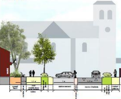
BB' COUPE DE PRINCIPE SUR LE MAIL MODES DOUX ET LA RUE DU CHABLAIS Echelle : 1/100'
